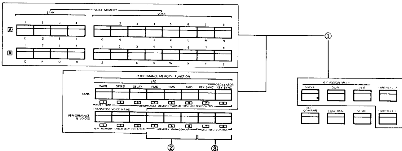
Fig. 55. Function Mode Parameter Switches
